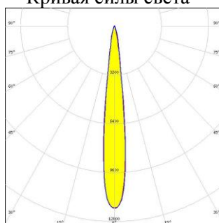
Кривая силы света
